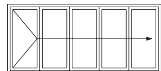
5-teiliges Element mit Drehflügel und vier Faltflügeln
